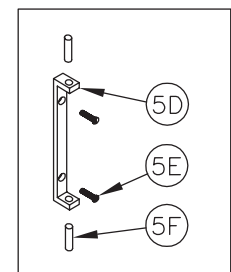
DETAIL: CLEANOUT DOOR HINGE 5D-F
